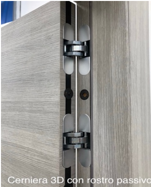
Cerniera 3D con rostro passivo
